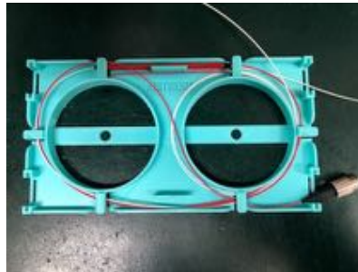
右側のファイバー巻き取り方法（下方）
